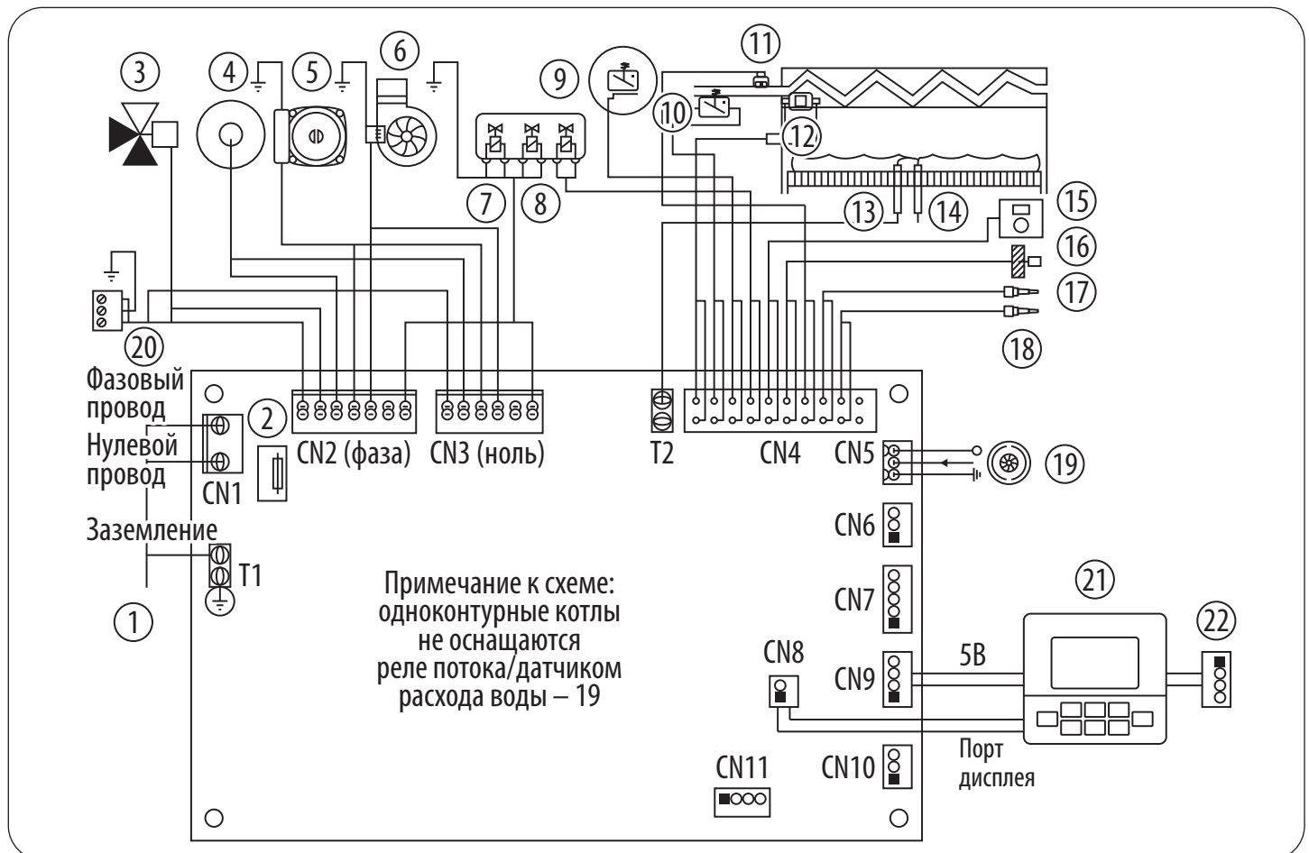
Рис. 46. Электрическая схема.
