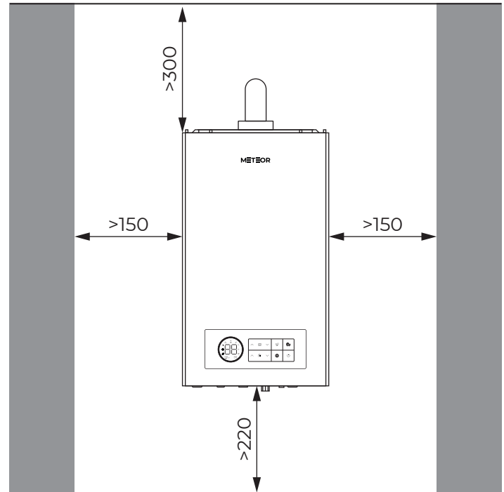
Рис. 44. Рекомендуемые расстояния для монтажа.
