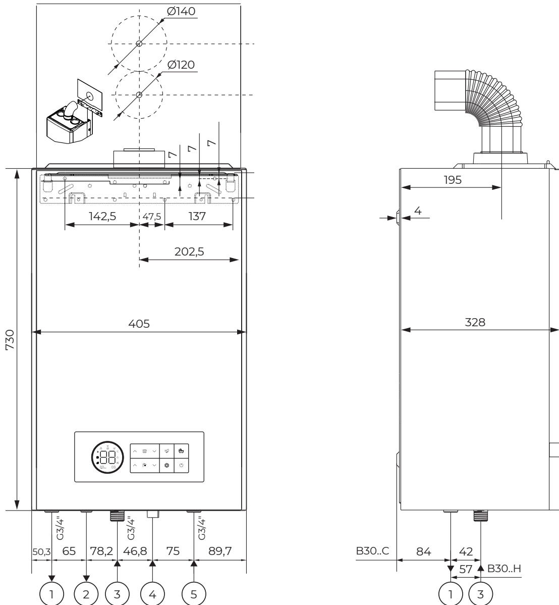
Рис. 43. В30 28 С/Н, В30 32 С/Н, В30 36 С/Н.
