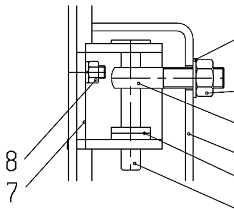
Рис. 4: Верхняя шарнирная группа со стороны открывания
