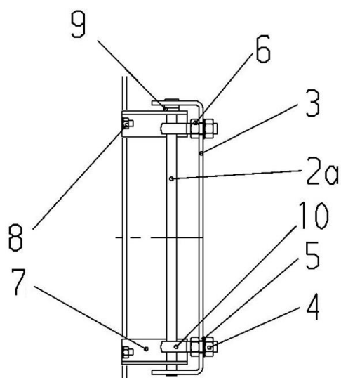
Рис. 1. Шарнирная группа на стороне упора
