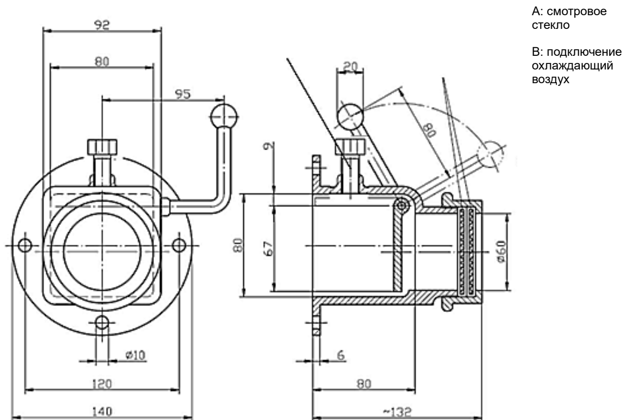
Рис. 12: Особенность смотрового отверстия факела, диаметр 60 мм
