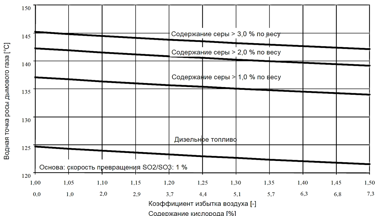
Диаграмма 2: Кислотная точка росы дымового газа при сгорании различных видов топлива (дизельное топливо; мазут с содержанием серы 1,0% по весу; мазуты с высоким содержанием серы: кислотная точка росы на основании содержания серы).
