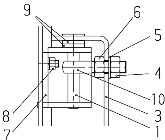
Рис. 3: Шарнирная группа на стороне упора
