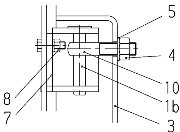
Рис. 7: Верхняя шарнирная группа со стороны открывания
