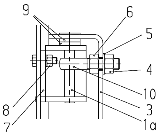
Рис. 6: Шарнирная группа на стороне упора
