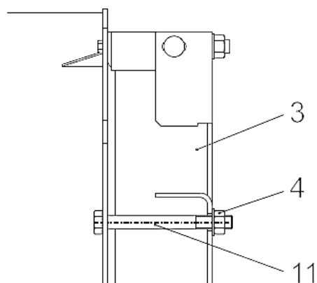
Рис. 10: Детали нажимной группы
