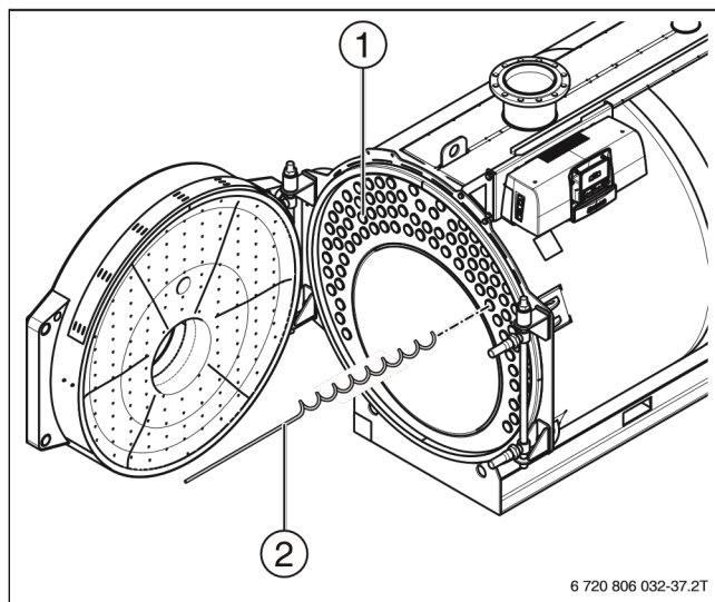
Рисунок 22 Удаление турбулизаторов
