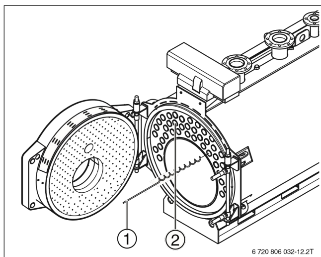
Рисунок 25 Корректировка предварительного натяжения турбулизаторов
