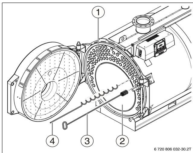
Рисунок 23 Чистка поверхностей нагрева
