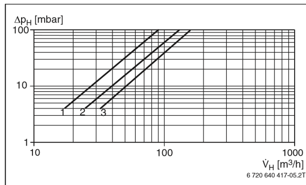
Рисунок 7 Гидравлическое сопротивление котлов SK 730 - 1850 кВт
