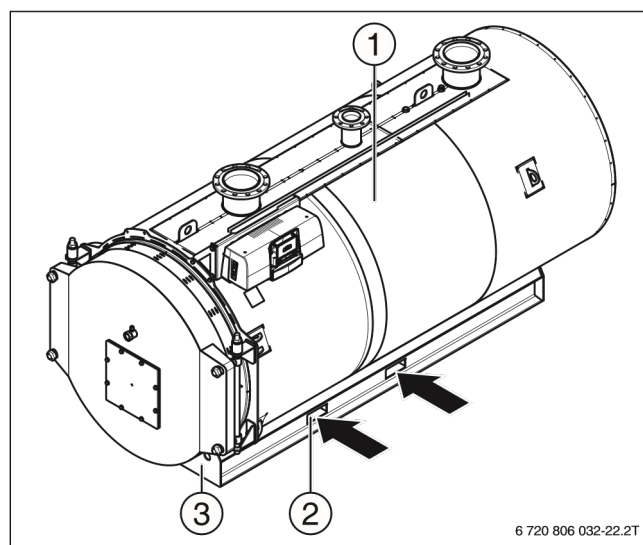
Рисунок 8 Транспортировка котла вилочным погрузчиком
