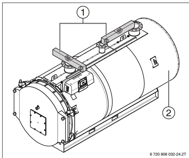
Рисунок 12 Выравнивание котла
