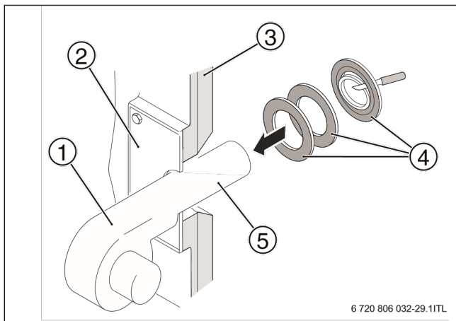
Рисунок 19 Монтаж горелки
