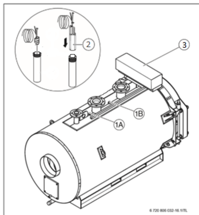
Рисунок 20 Установка датчика температуры SK 120 – 820 кВт
